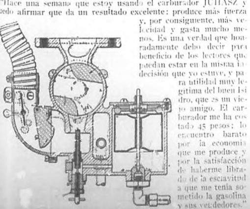
Diseño del carburador "JUHASZ".
